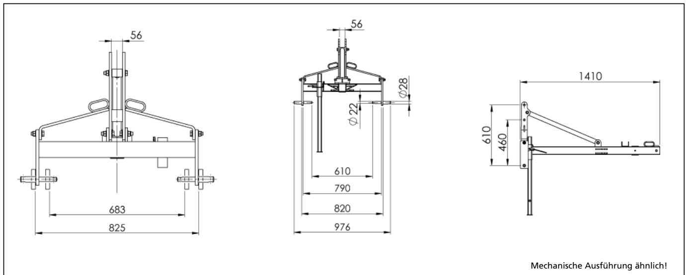
Dreipunktbock: KAT I / II
