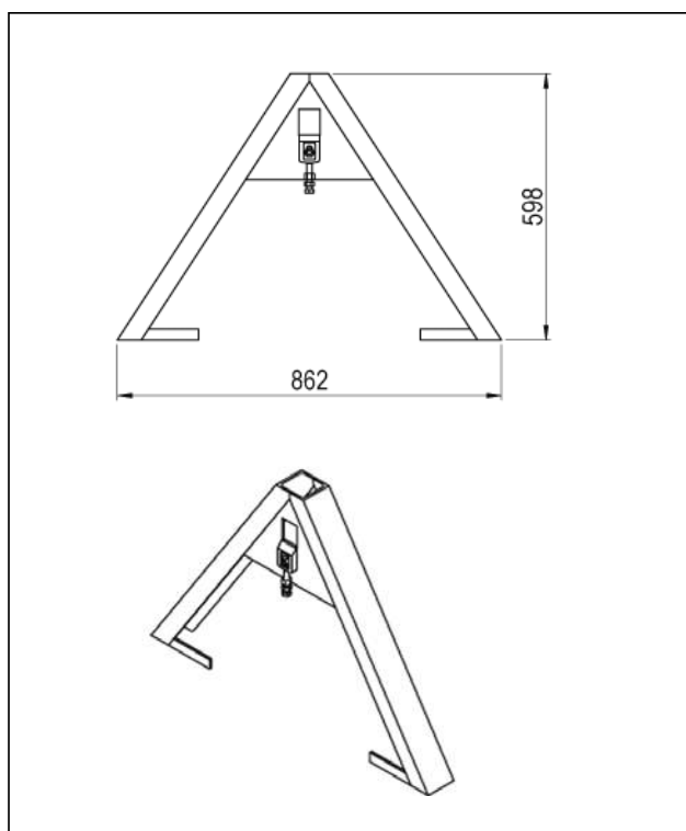
Gerätedreieck: KAT I
