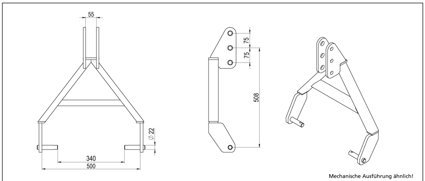
Dreipunktbock: KAT I N
